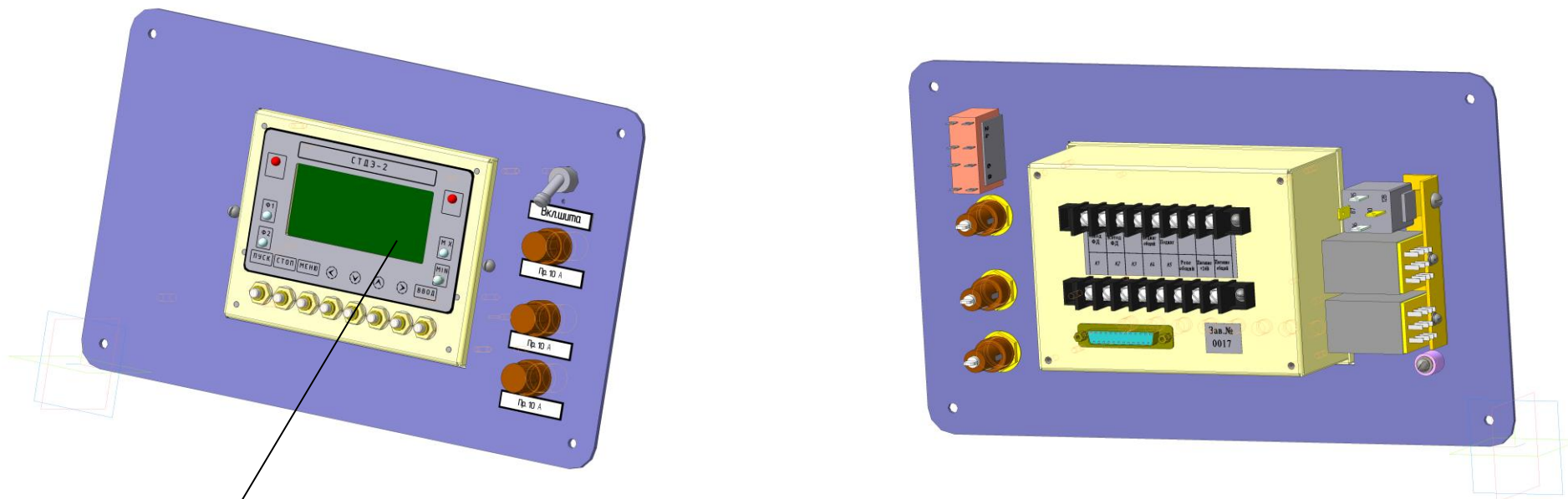
Блок управления и сигнализации БУС СТДЭ-2
